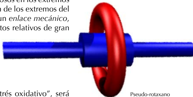
Pseudo-rotaxano
