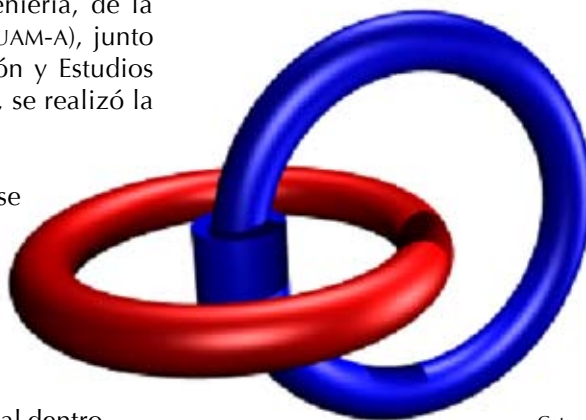
Catenano
